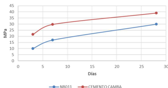
RESISTENCIA DE CEMENTO CAMBA IF-30
